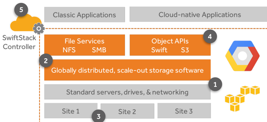
Anatomy of SwiftStack Object Storage.
