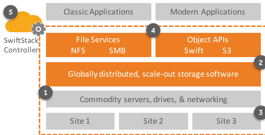
Anatomy of SwiftStack Object Storage.
